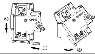
TH35-7.5 DIN Rail
